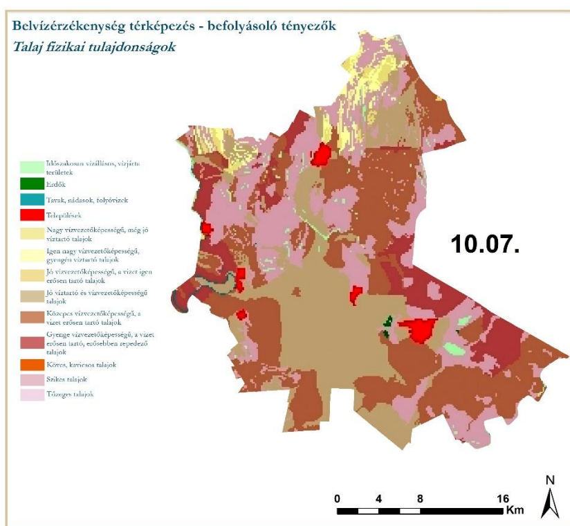
14. ábra: Talajtani környezeti segédváltozó – Talajfizika
