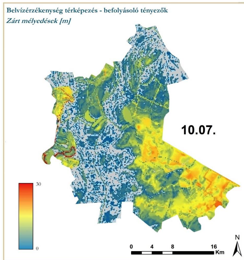
9. ábra: Domborzati környezeti segédváltozó – Zárt mélyedések
