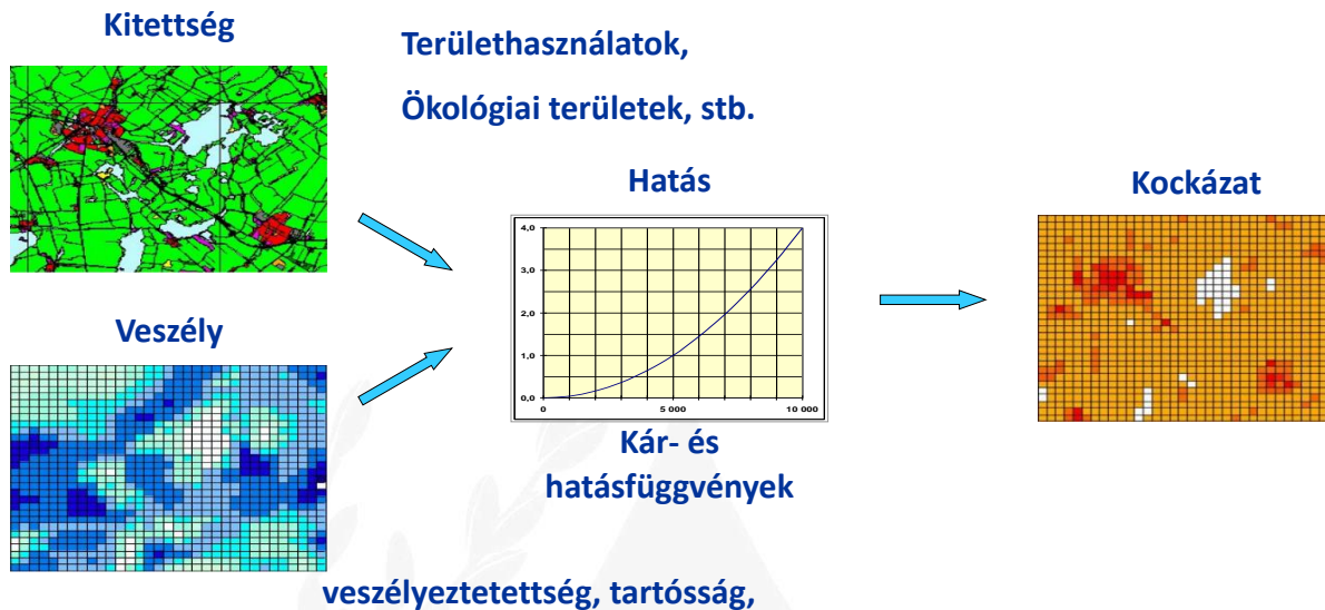
29.ábra: A kockázatszámítás tematikája
