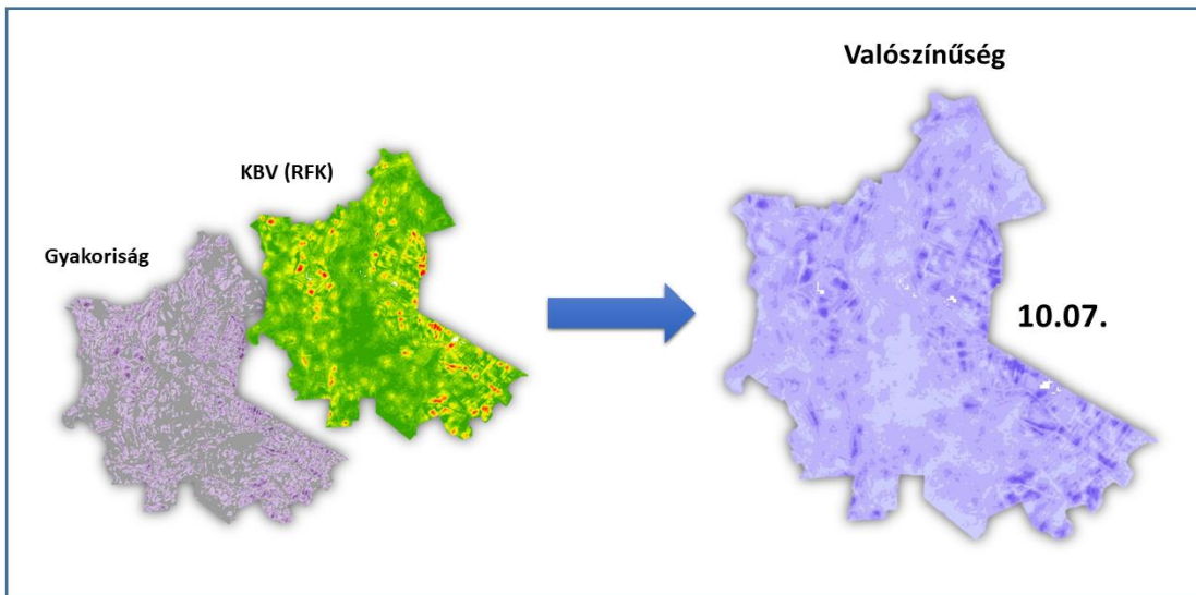
30.ábra: A valószínűségi térkép szerkesztése
