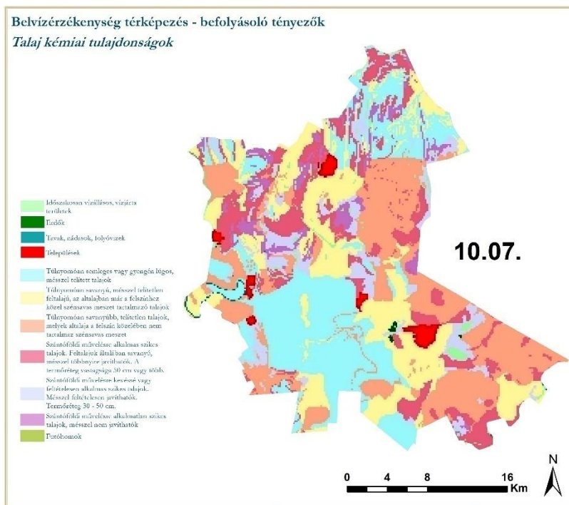
15. ábra: Talajtani környezeti segédváltozó – Talajkémia
