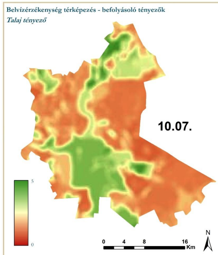
13.ábra: A talajtani tényező területi eloszlása
