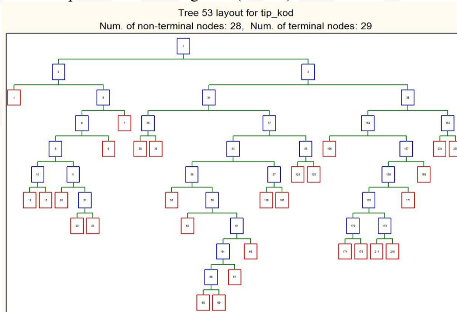
3. ábra: döntési fa
