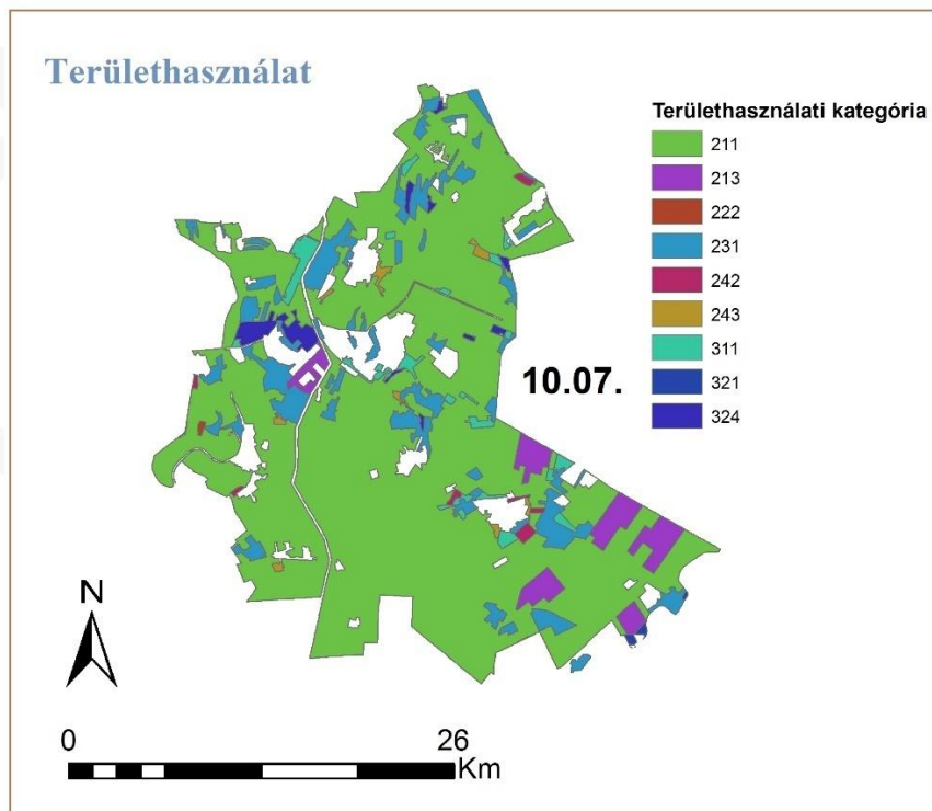
32.ábra: Az előfordulási valószínűség térképe
