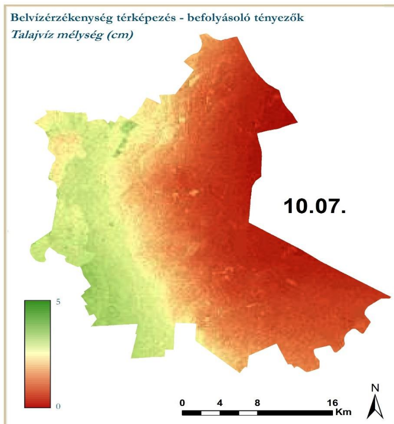
21. ábra: Ko-krigeléssel módosított talajvíz tényező térkép
