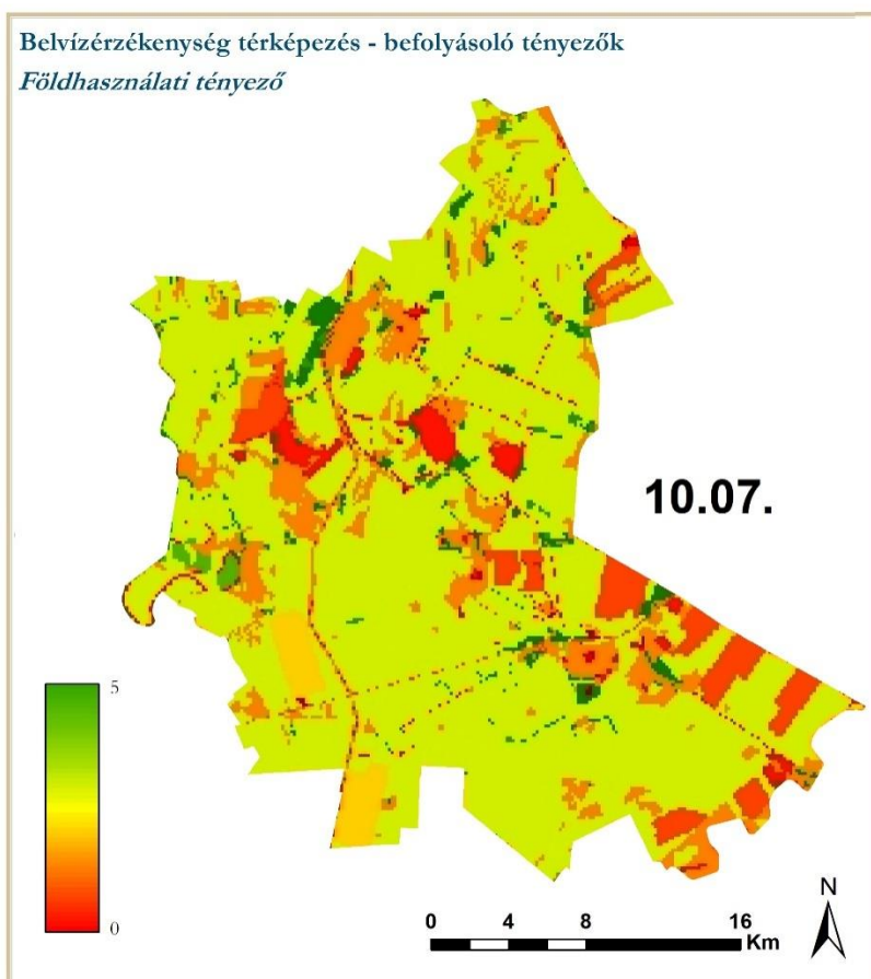
22. ábra: Földhasználati tényező térkép
