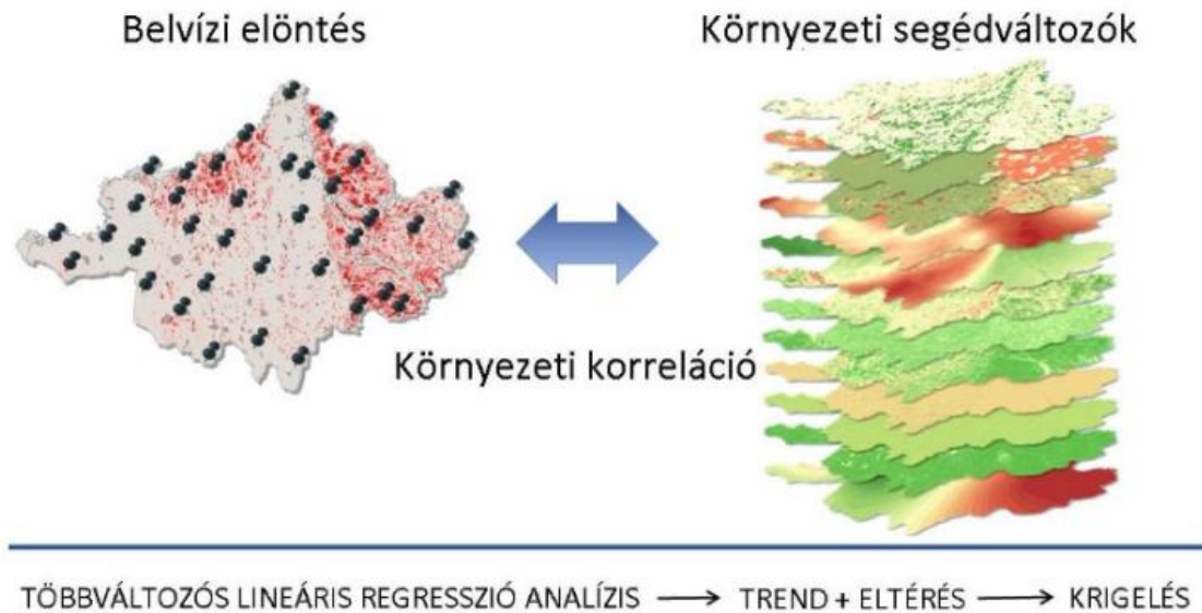
2. ábra: A regresszió krigelés menete
