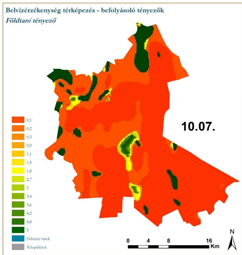
17. ábra: Földtani tényező térkép
