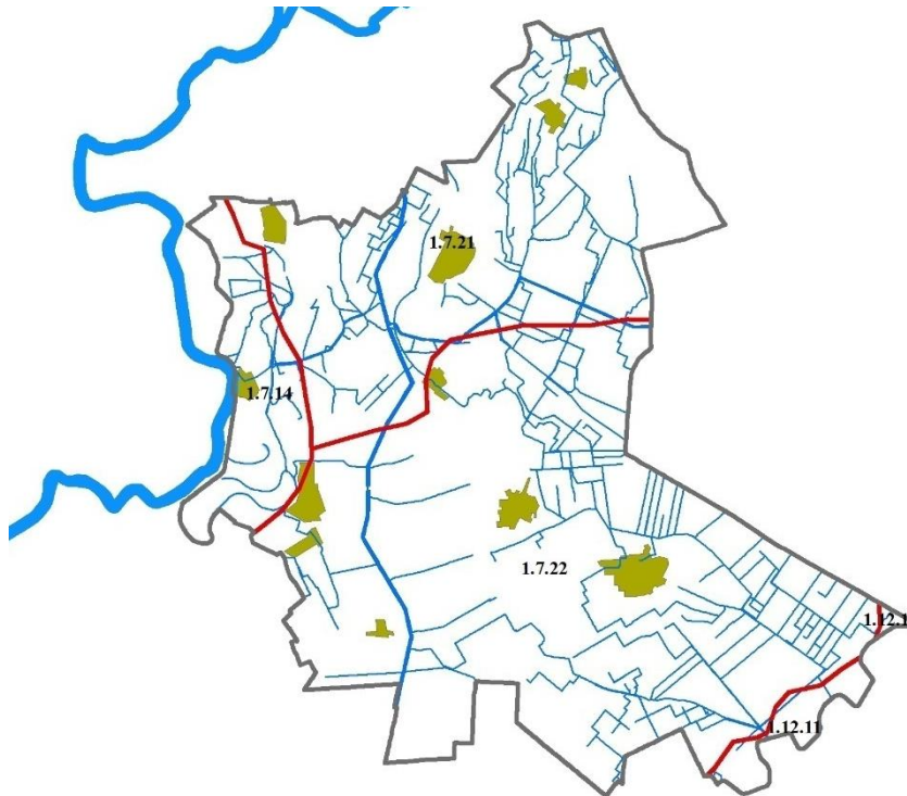
1.ábra: a 10.07. belvízvédelmi szakasz természetföldrajzi felosztása
