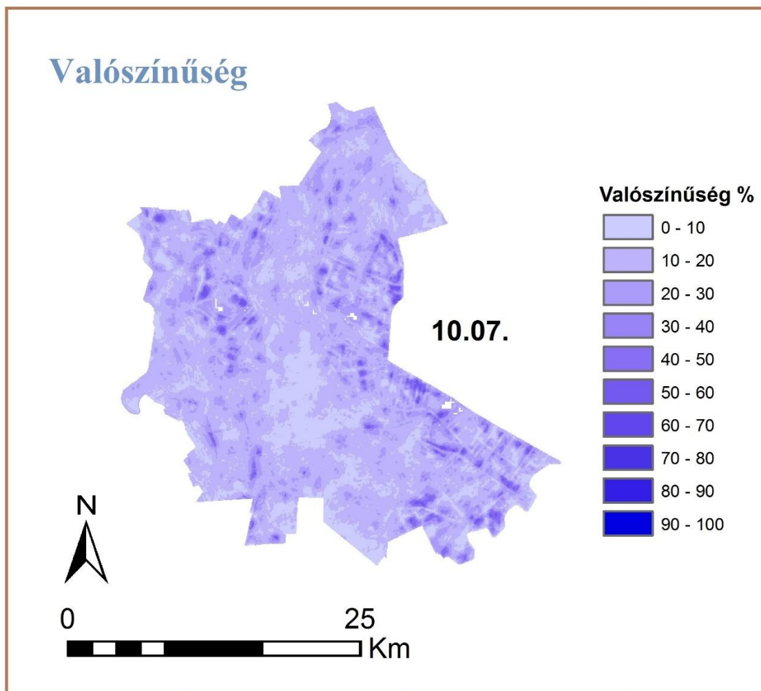
31.ábra: Az előfordulási valószínűség térképe
