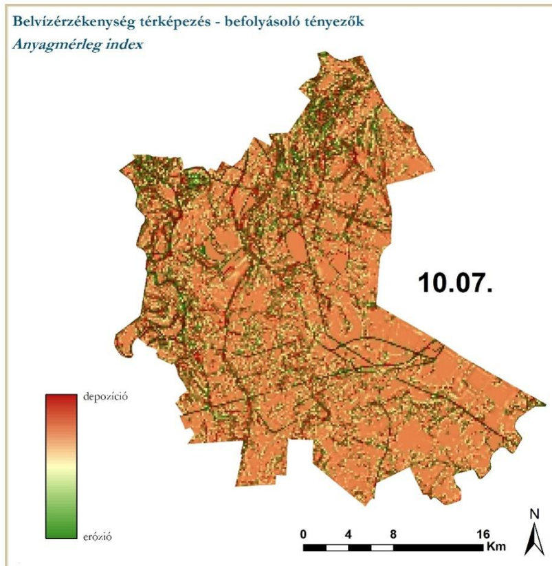
10ábra: Domborzati környezeti segédváltozó – Anyagmérleg index
