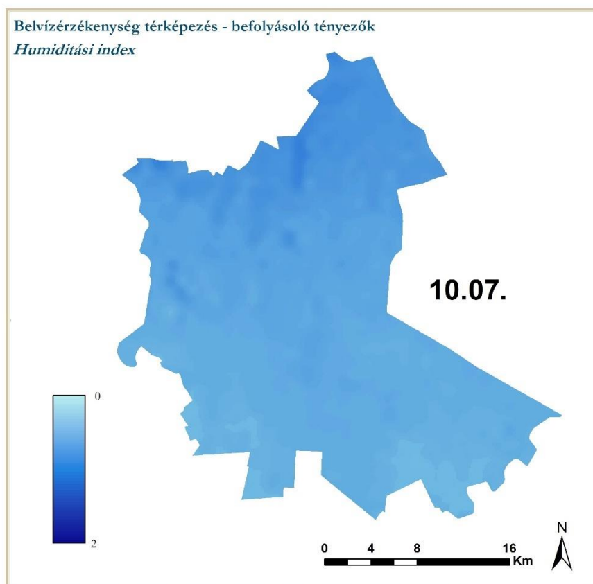
4. ábra: A hidrometeorológiai tényező területi eloszlása
