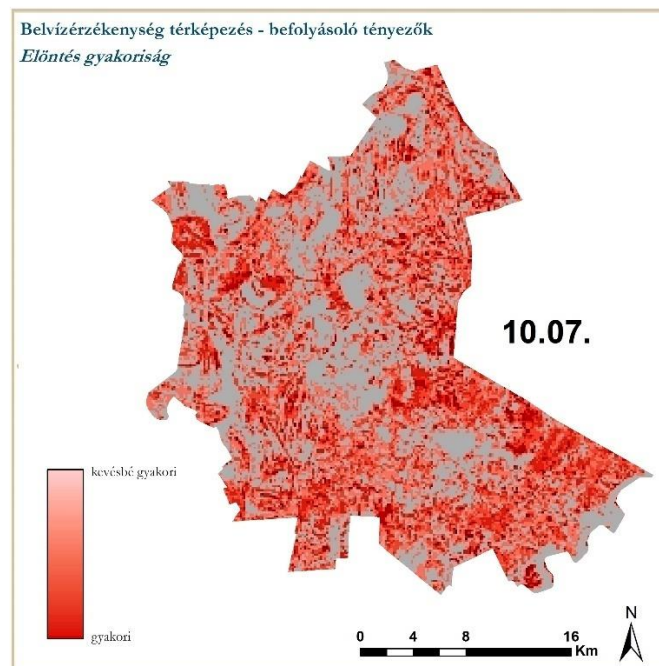
23. ábra: Belvív-gyakorisági térkép
