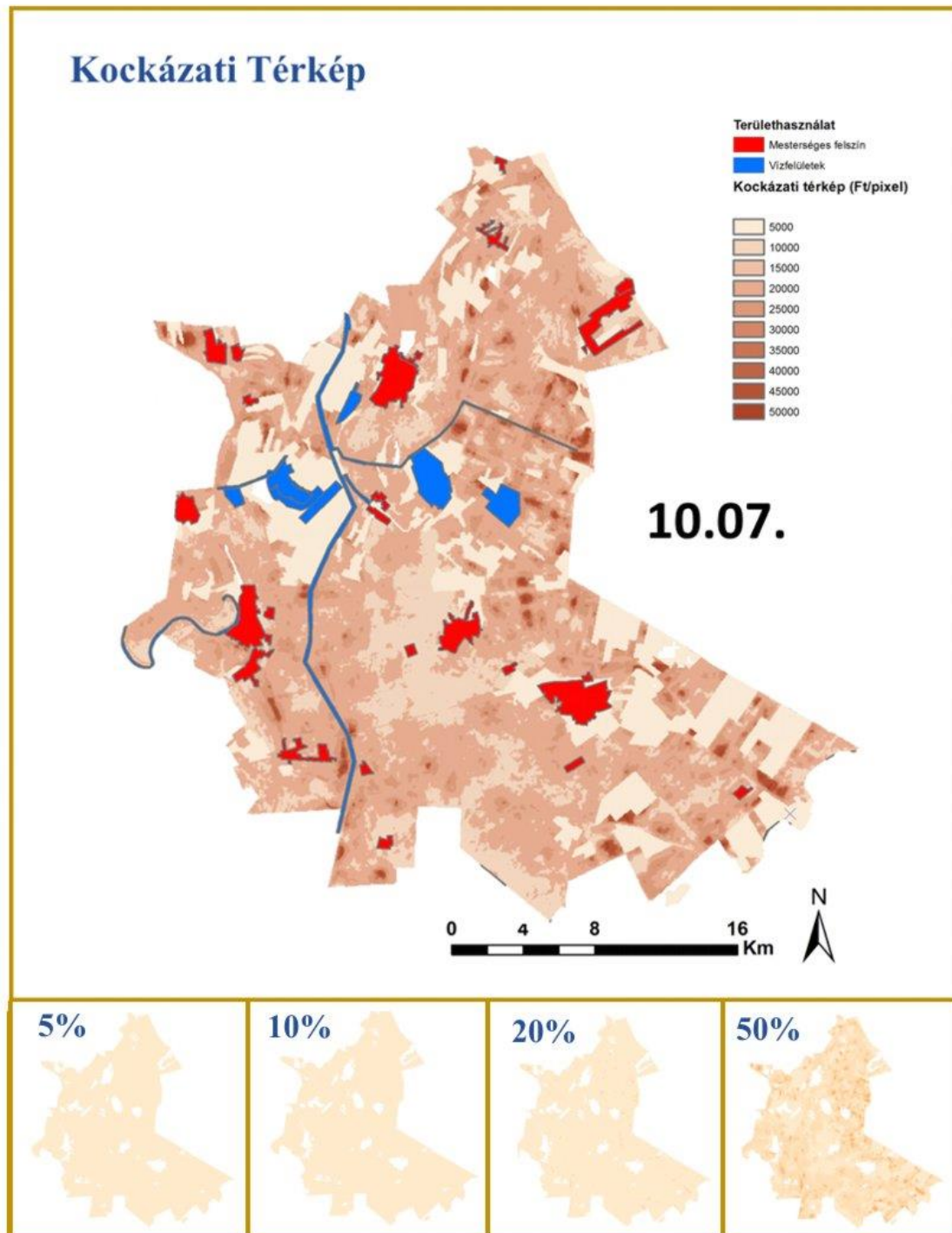
29.ábra: Az előfordulási valószínűség térképe
