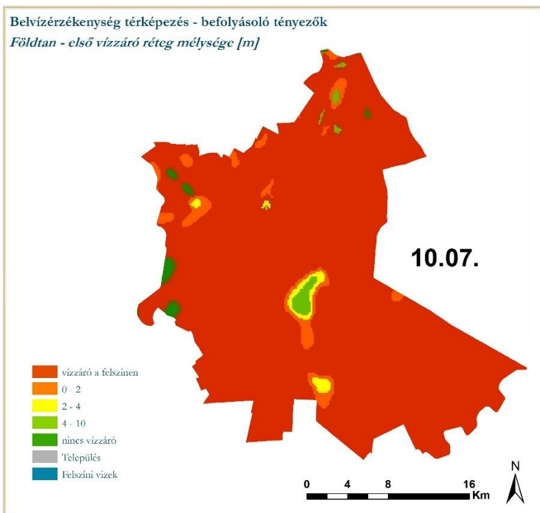
18. ábra: Sekélyföldtani környezeti segédváltozó – első vízzáró réteg mélysége (m)
