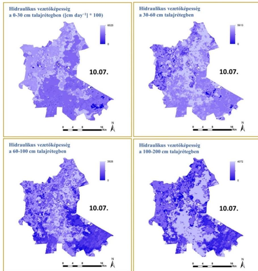
27. ábra: Talaj hidrofizikai tényezők II.
