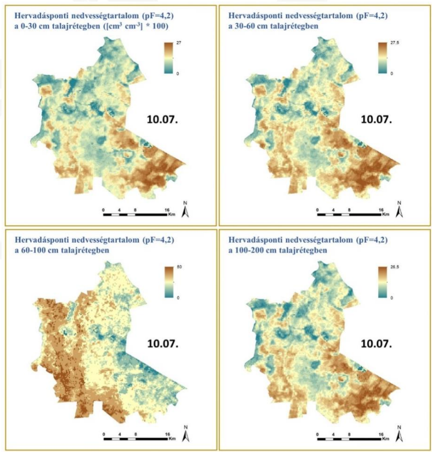
26. ábra: talaj hidrofizikai tényezők I.
