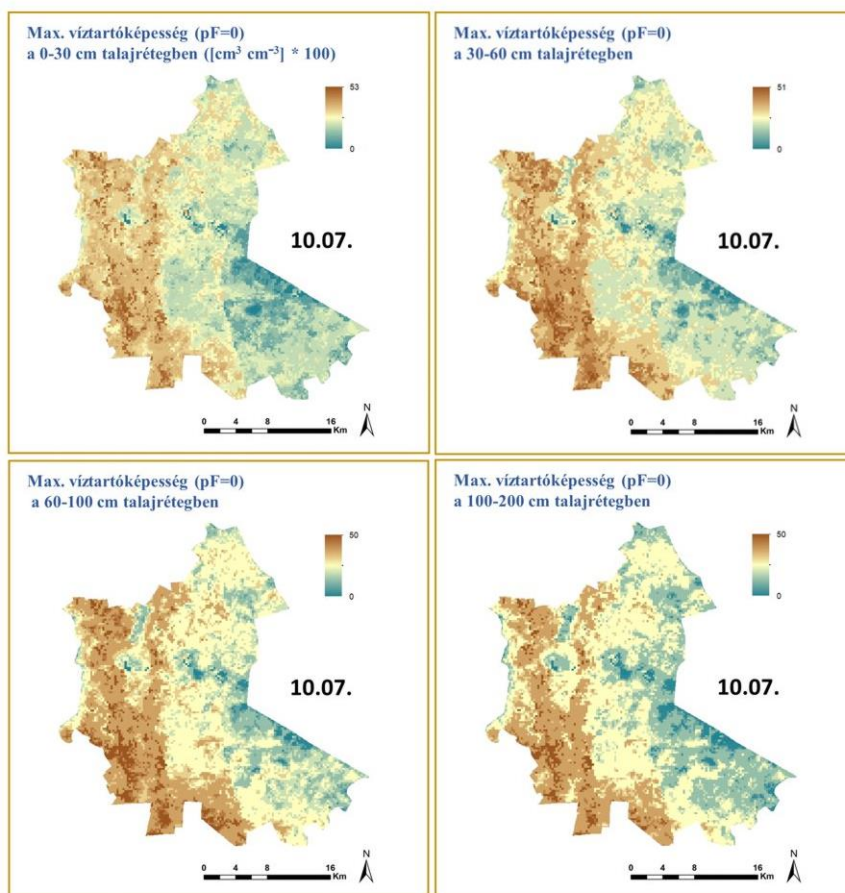
25. ábra: Hidrológiai és hidromorfológiai tényezők
