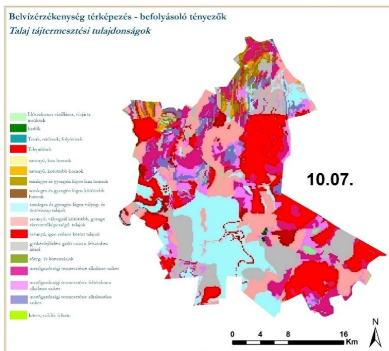
16. ábra: Talajtani környezeti segédváltozó – Tájtermesztési tulajdonságok
